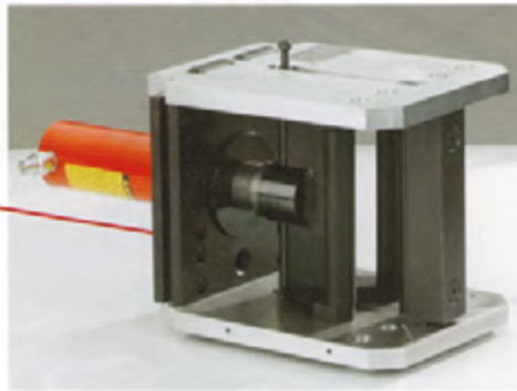
"V" bockning
